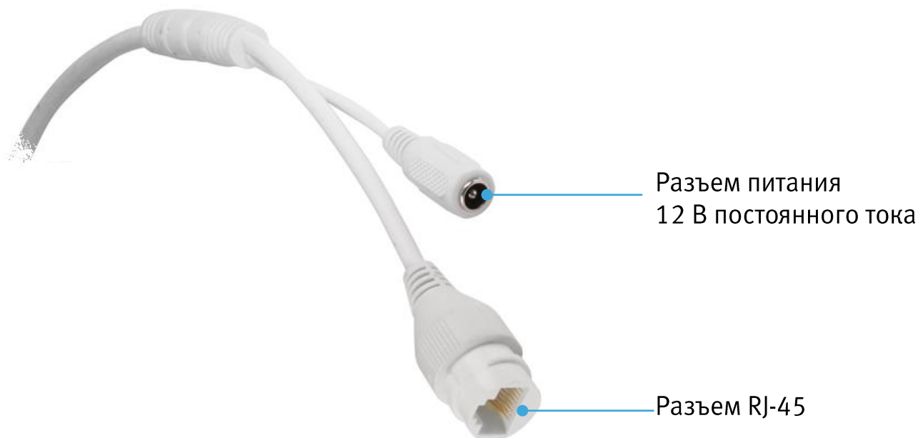
Рисунок 6.1 – Кабель видеокамеры
