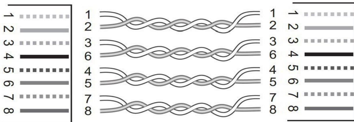
Схема подсоединения проводов при наличии расщепленных пар
