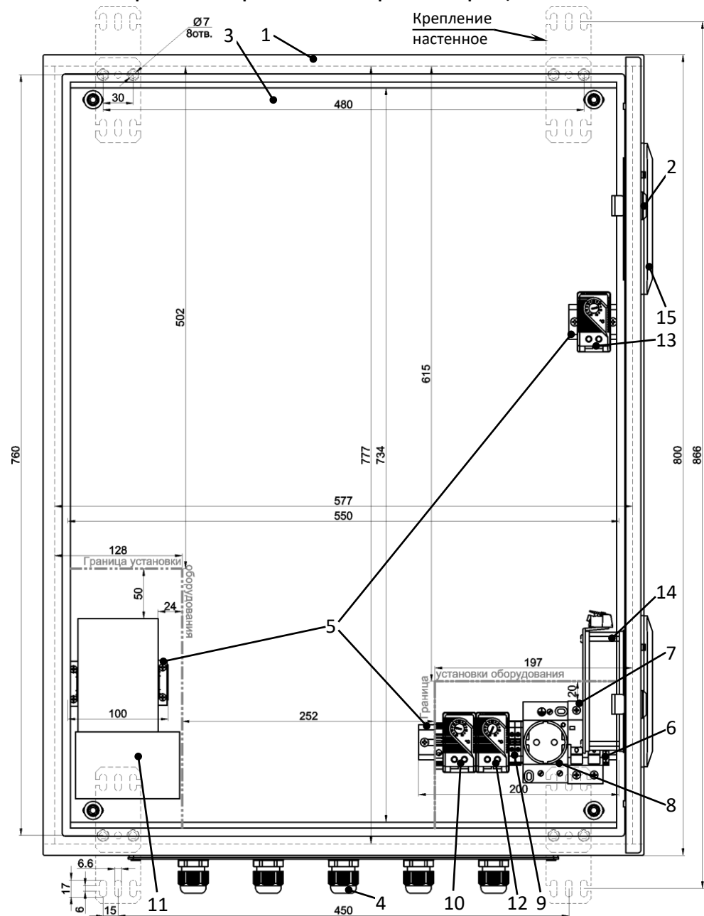
Рисунок 1 – Устройство шкафа
