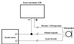
Схема подключения электрическая
