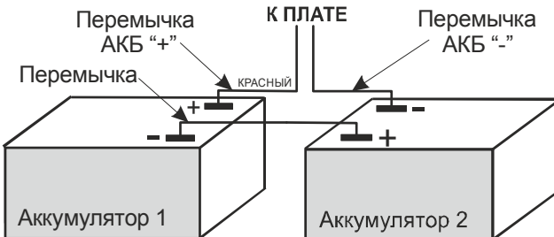
Рисунок 3 – подключение АКБ
