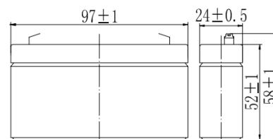
Габариты
