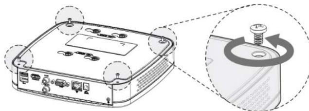
Рисунок 3.3 – Установка жесткого диска
