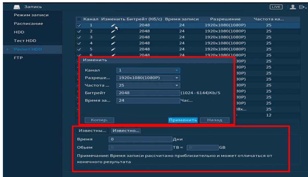
Рисунок 6.70 – Расчет объема
