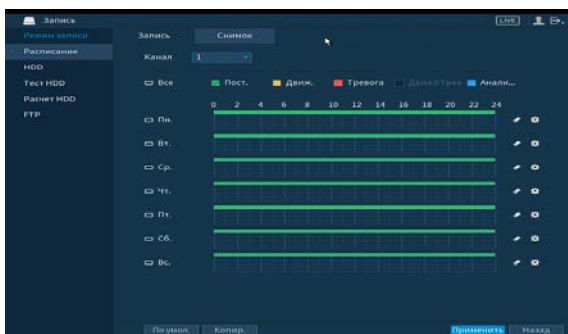
Рисунок 6.64 – Настройка расписания
