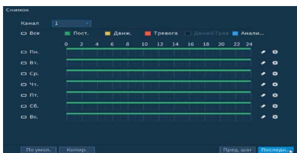
Рисунок 4.18 – Настройка расписания
