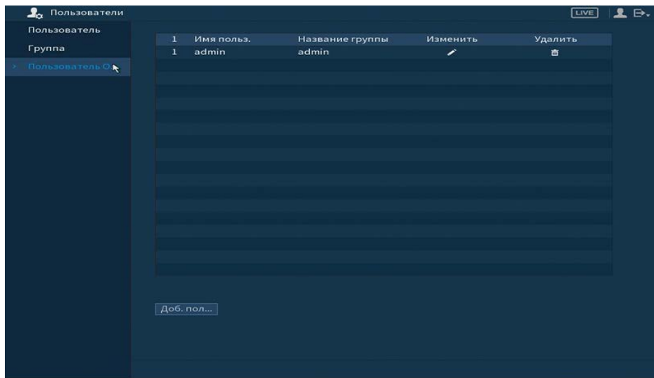
Рисунок 6.91 – Настройка ONVIF
