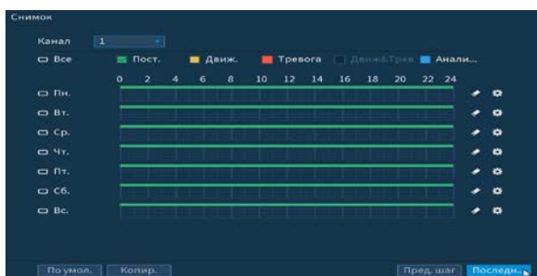
Рисунок 4.15 – Настройка расписания
