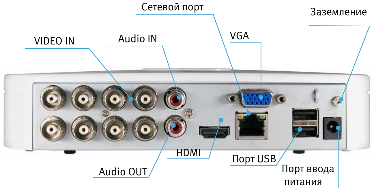
Рисунок 3.2 – Внешний вид задней панели
