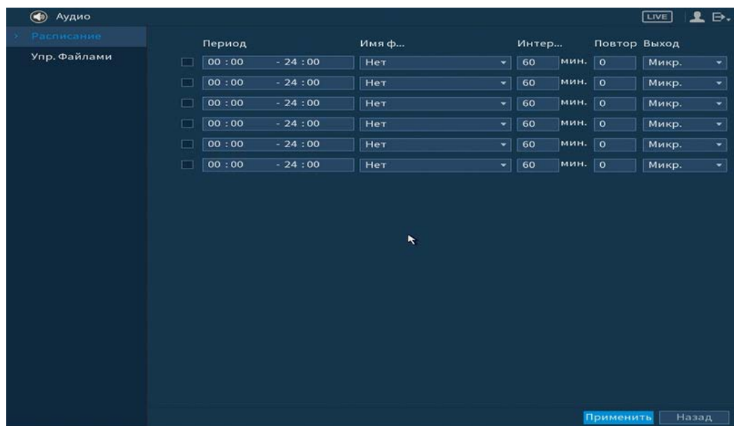
Рисунок 6.30 – Установка расписания
