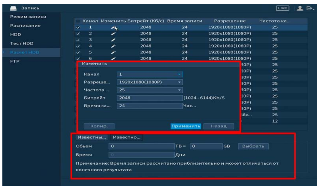
Рисунок 6.69 – Расчет времени
