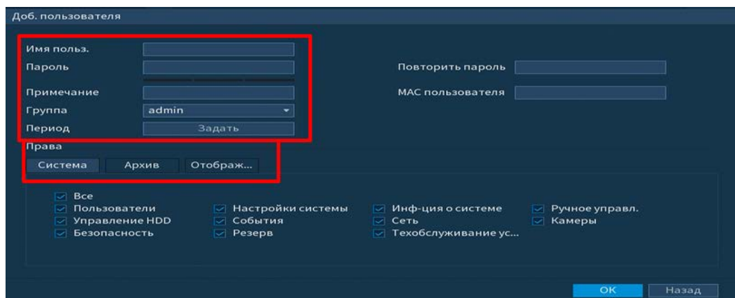
Рисунок 6.88 – Добавление пользователя
