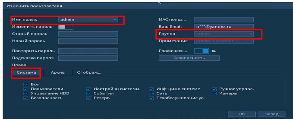
Рисунок 6.87 – Назначение прав
