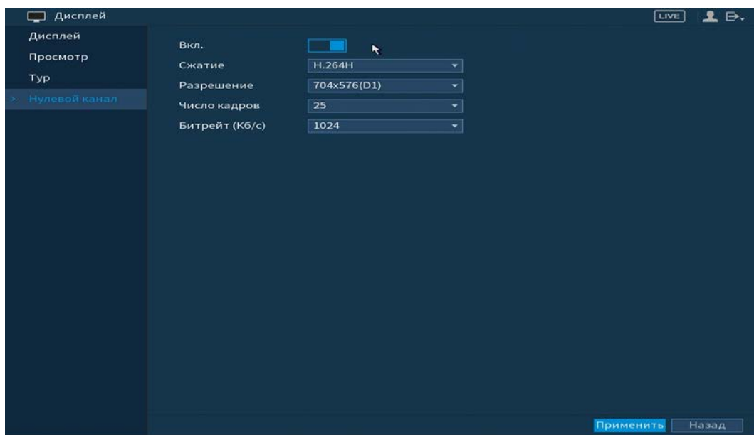
Рисунок 6.29 – Интерфейс настройки
