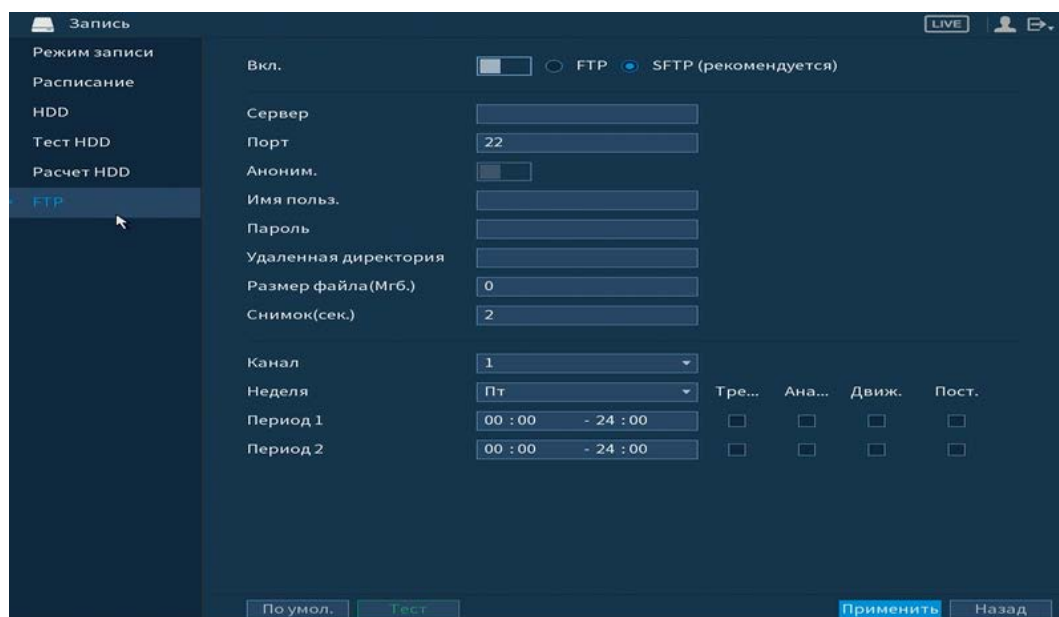
Рисунок 6.71 – Настройка FTP
