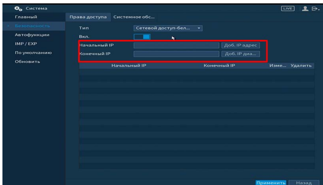
Рисунок 6.75 – Права доступа
