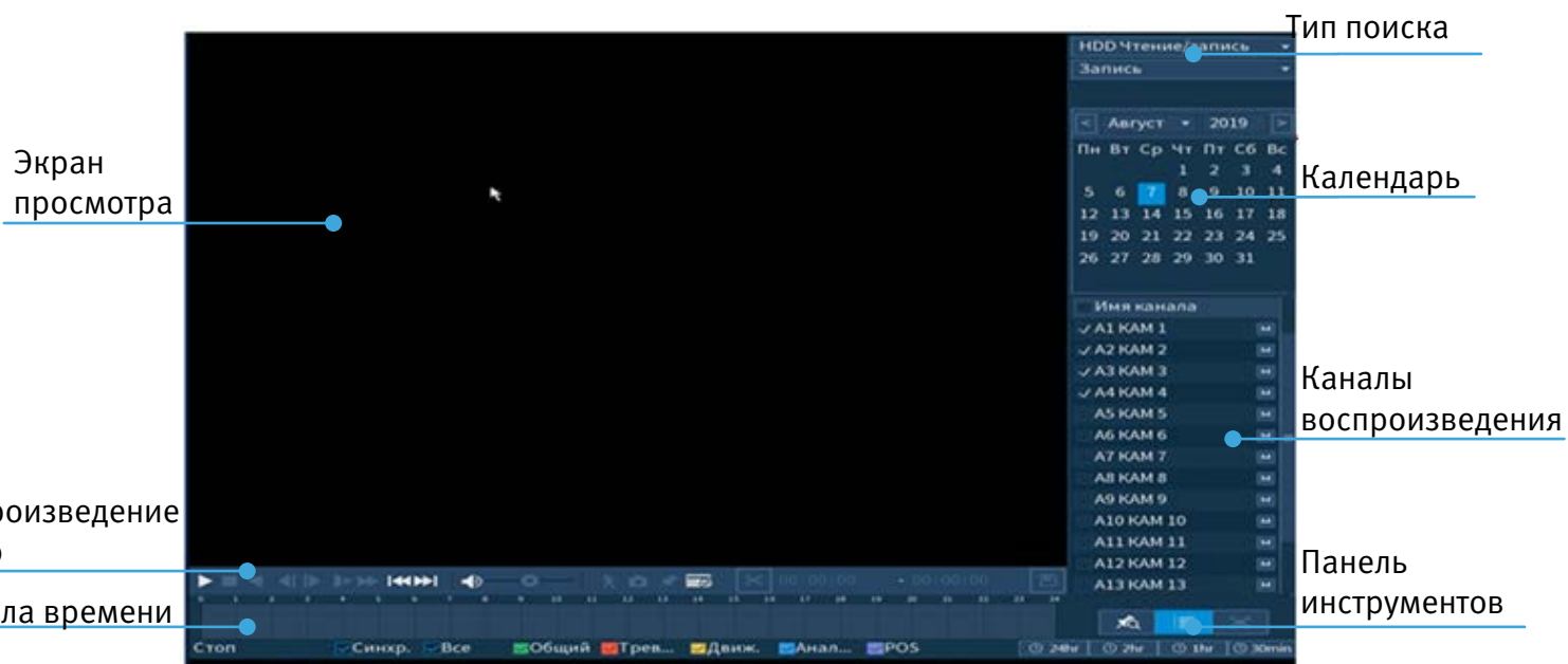
Рисунок 6.2 – Просмотр архива
