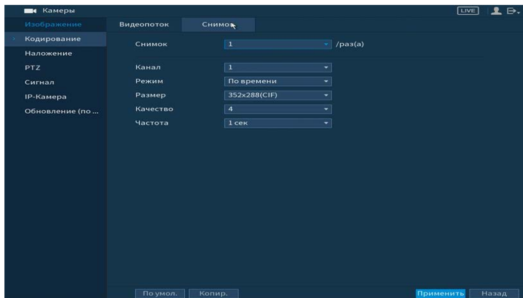
Рисунок 6.35 – Настройка снимка
