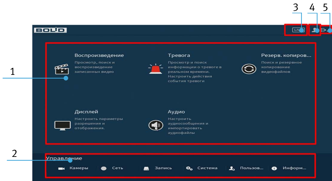
Рисунок 6.1 – Главное меню
