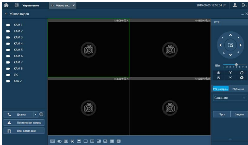
Рисунок 10.2 – Режим просмотра
