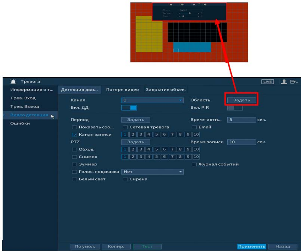
Рисунок 6.18 – Настройка области
