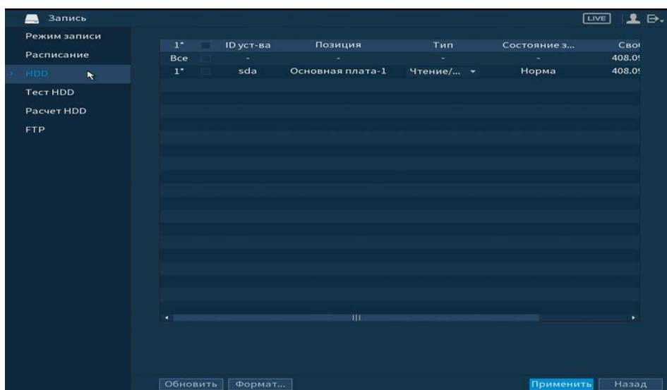
Рисунок 6.66 – Интерфейс настройки
