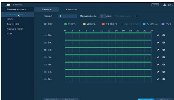
Рисунок 6.61 – Настройка расписания
