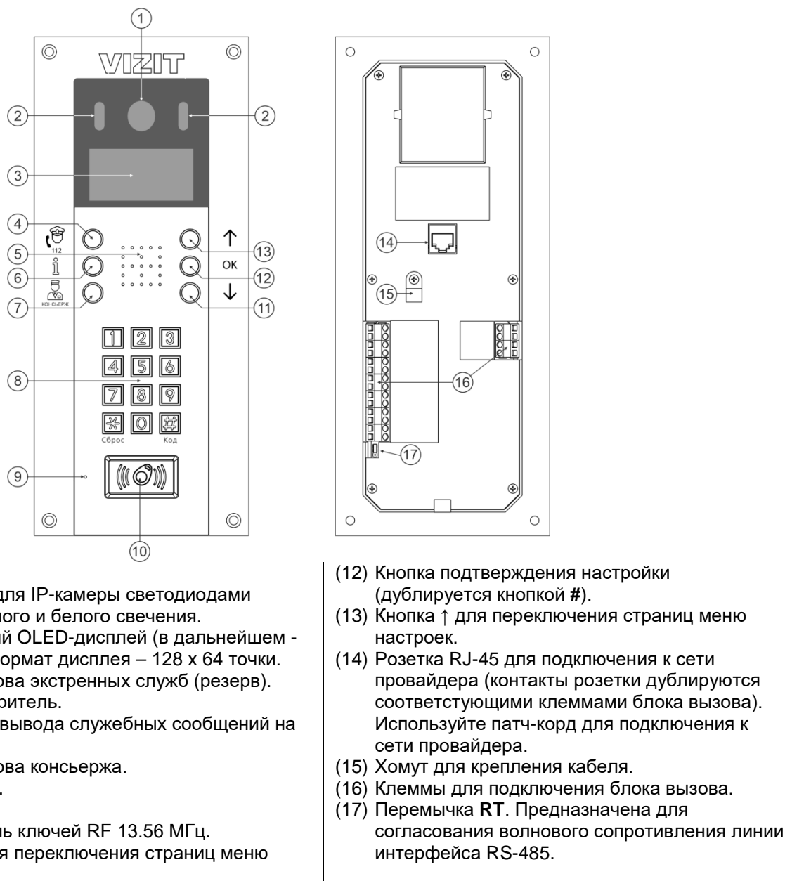
Рисунок 2.1 - Внешний вид блока вызова
