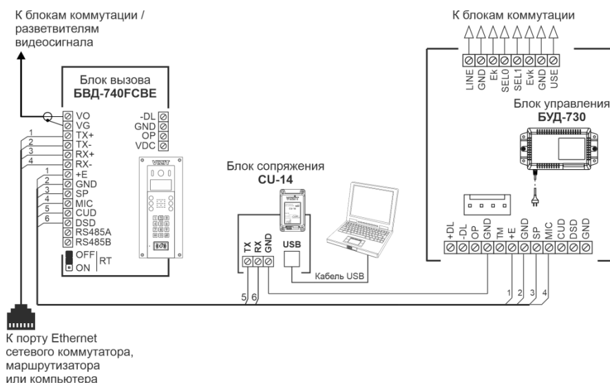
Рисунок 17.1 - Схема соединений блока вызова с блоком управления БУД-730 и блоком сопряжения CU-14
